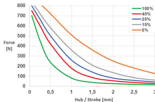
Kraft / Weg-Kennlinie Kühlblech
